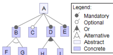
Fig. 1. Modelo de Características
